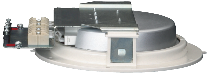
Abb.: Decken-Einbauleuchte P 03 Höhe 51 mm
