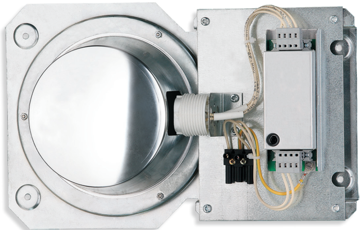
Abb.: Decken-Einbauleuchte, rund 00 92 50 Ansicht von hinten
