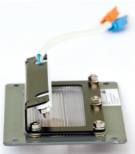
Abb.: LED-Trittstufenleuchte 143 567_96 Ansicht von hinten
